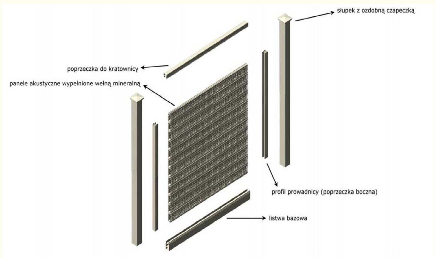
Rys. 3 Schemat budowy płotu akustycznego w opcji bez kratownicy.
