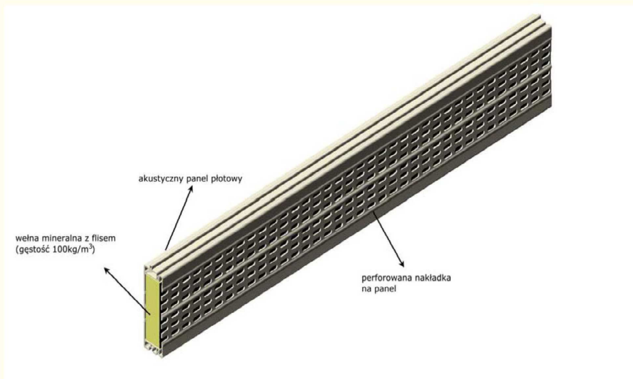
Rys. 4 Schemat budowy panelu akustycznego.
