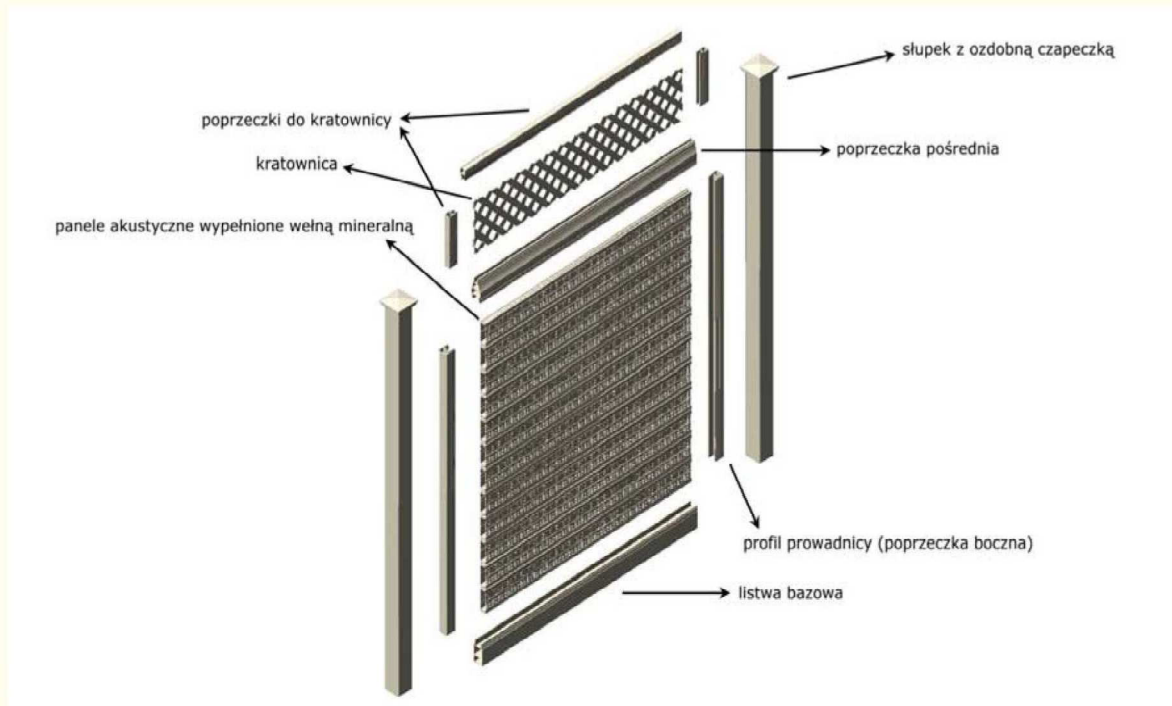
Rys. 2 Schemat budowy płotu akustycznego w opcji z kratownicą.
