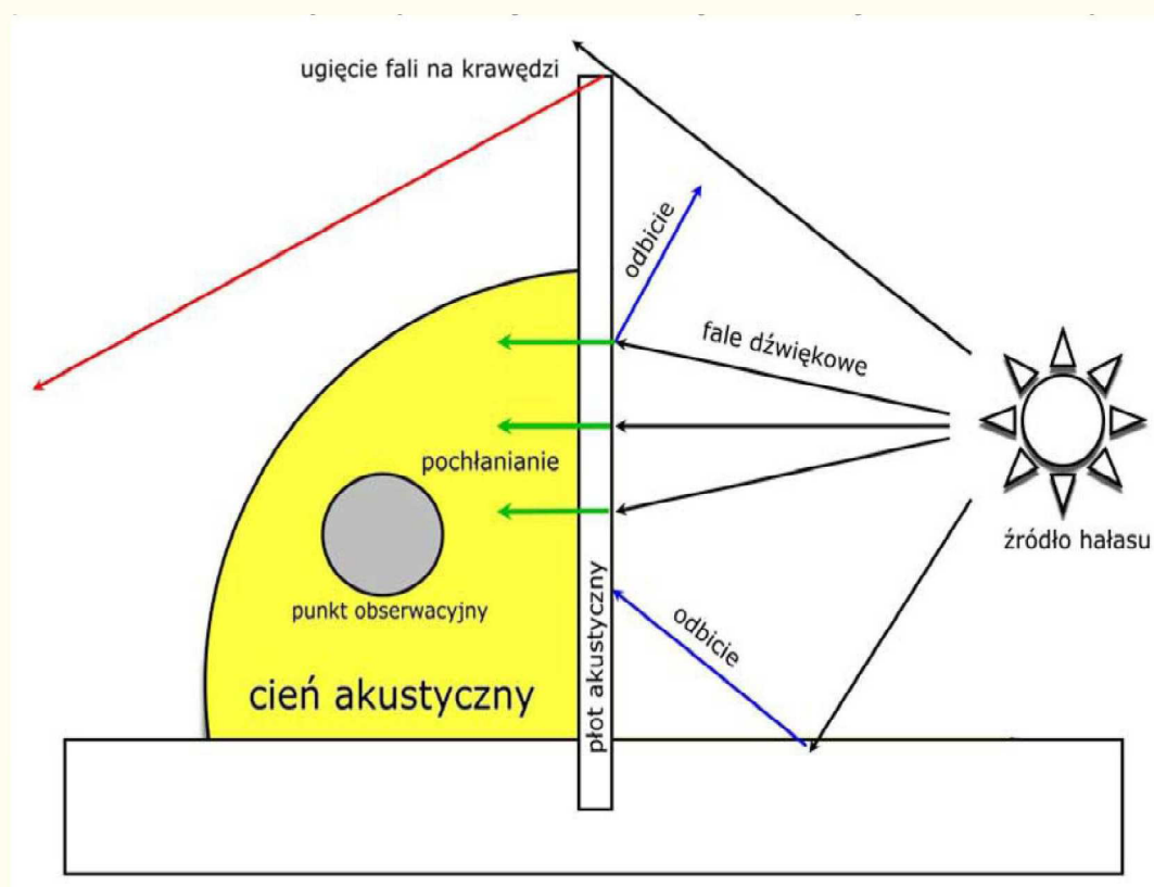
Rys.1 Sposób działania płotu akustycznego.
